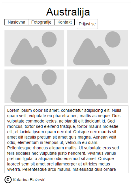
Slika 3. Izgled mrežne stranice na mobilnom uređaju
