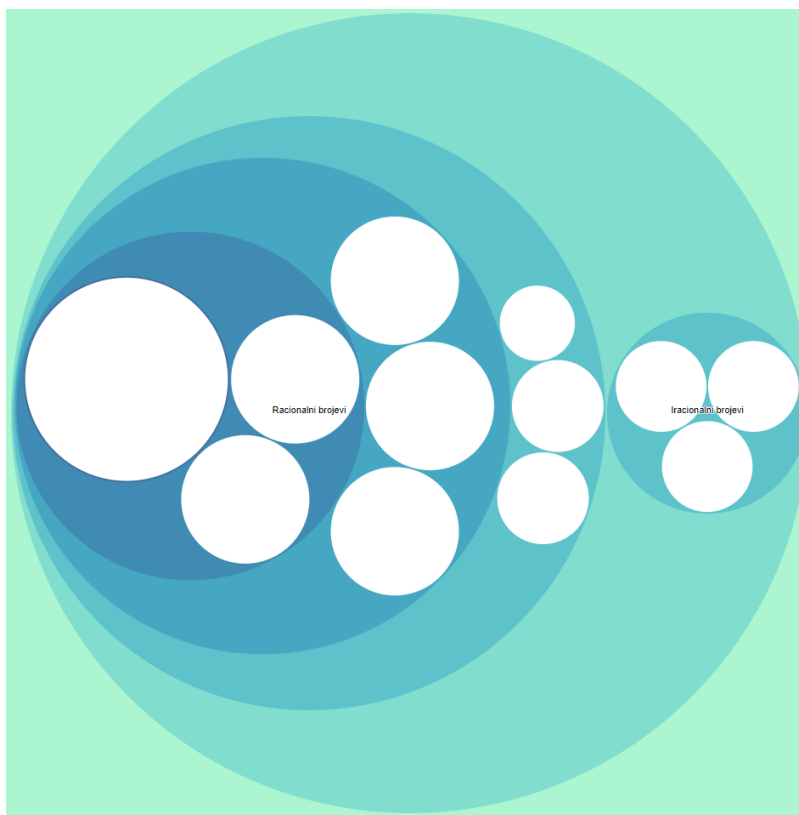
Slika 10. Vizualni prikaz skupa realnih brojeva
