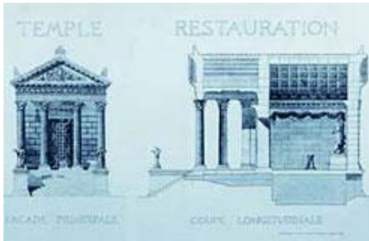
Prilog 50: Pročelje i presjek malog hrama Dioklecijanove palače
