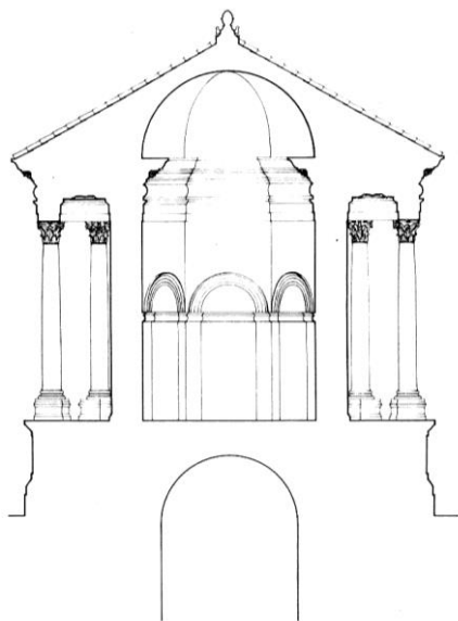
Prilog 53: Rekonstrukcija „Venerina“ hrama
