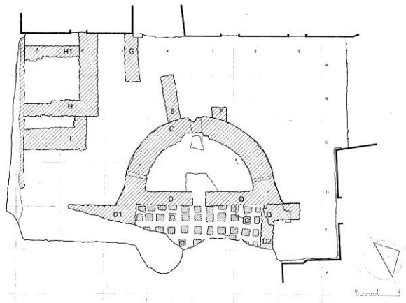
Prilog 39: Tlocrt istočnih termi
