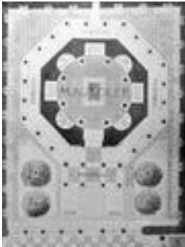
Prilog 47: Tlocrt Mauzoleja
