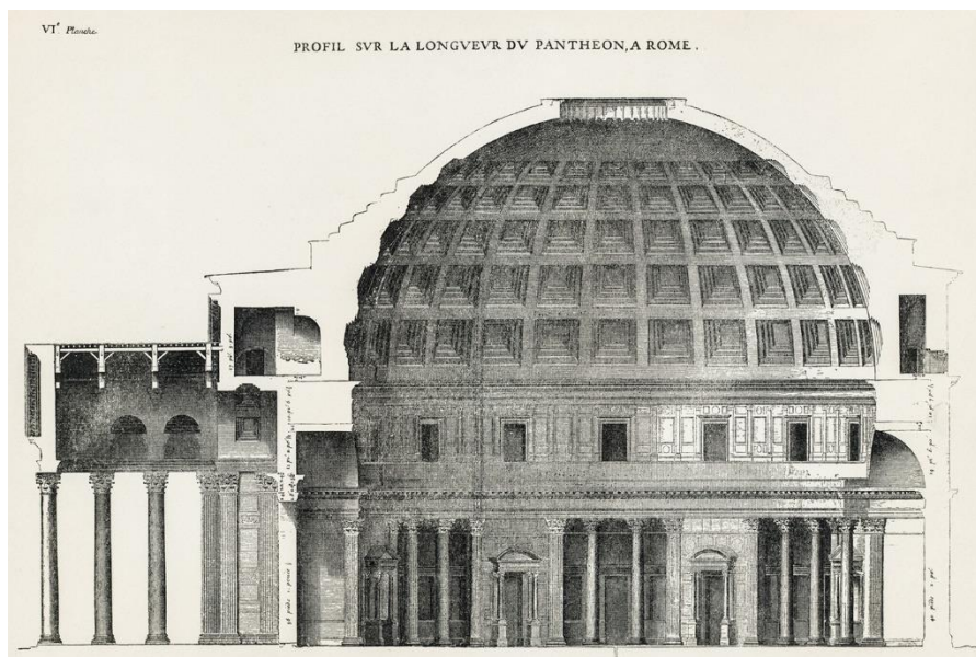
Slika 3. Presjek Panteona
