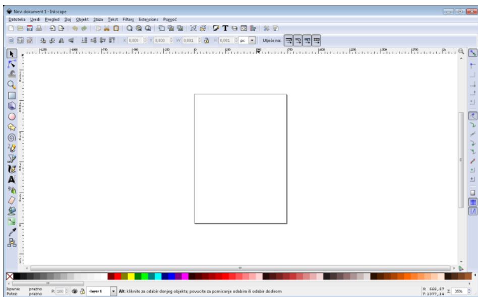
Slika 9. Inkscape - sučelje
