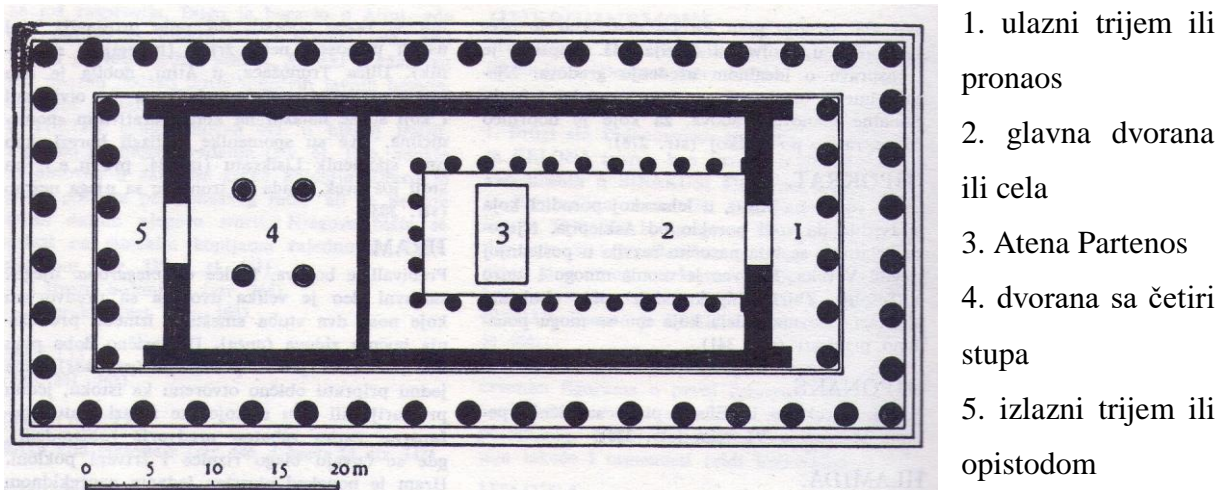
Slika 9. tlocrt Partenona
