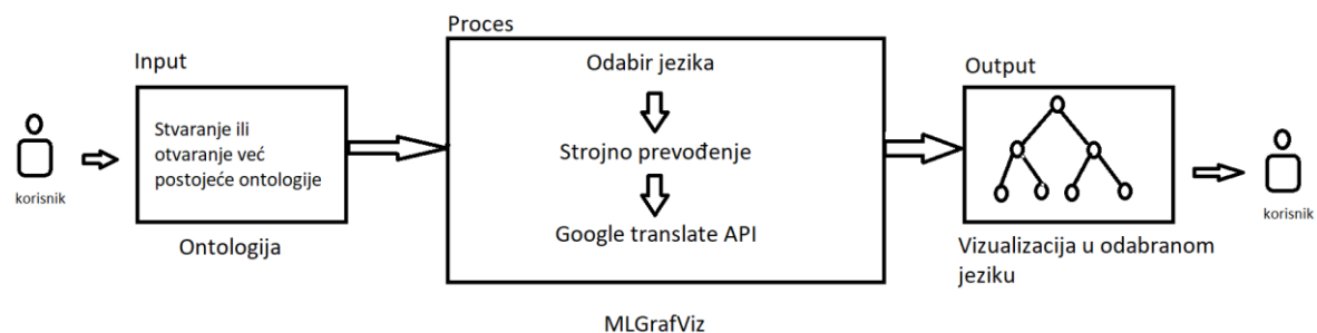
Slika 4. MLGrafViz funkcionalnost
