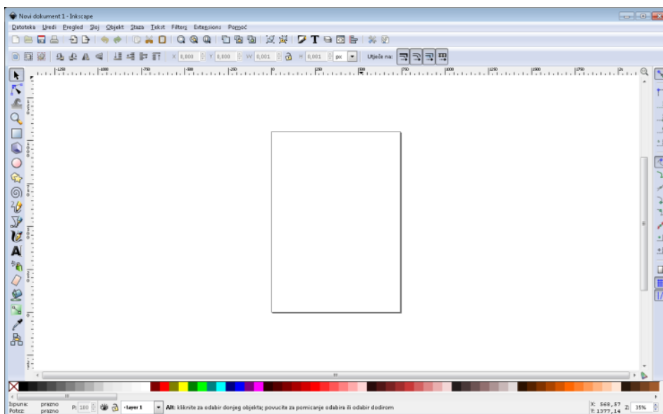
Slika 9. Inkscape - sučelje
