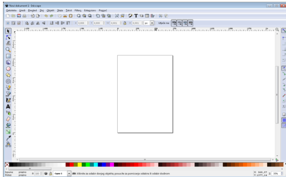
Slika 9. Inkscape - sučelje
