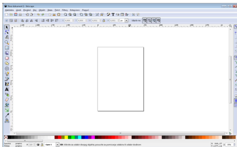
Slika 9. Inkscape - sučelje
