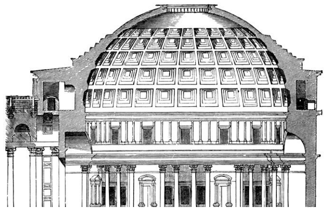
Slika 19: Presjek Panteona
