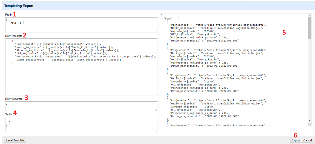
Slika 12 - Prozor za kreiranje predloška povezanih podataka.
