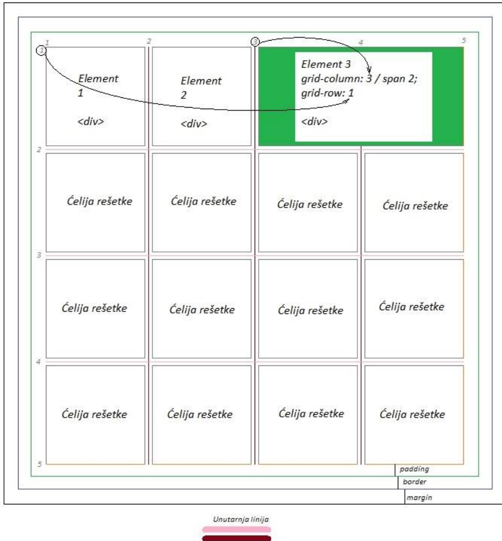
Slika 2: vizualna reprezentacija CSS box modela i osnova rada CSS rešetaka. 10
