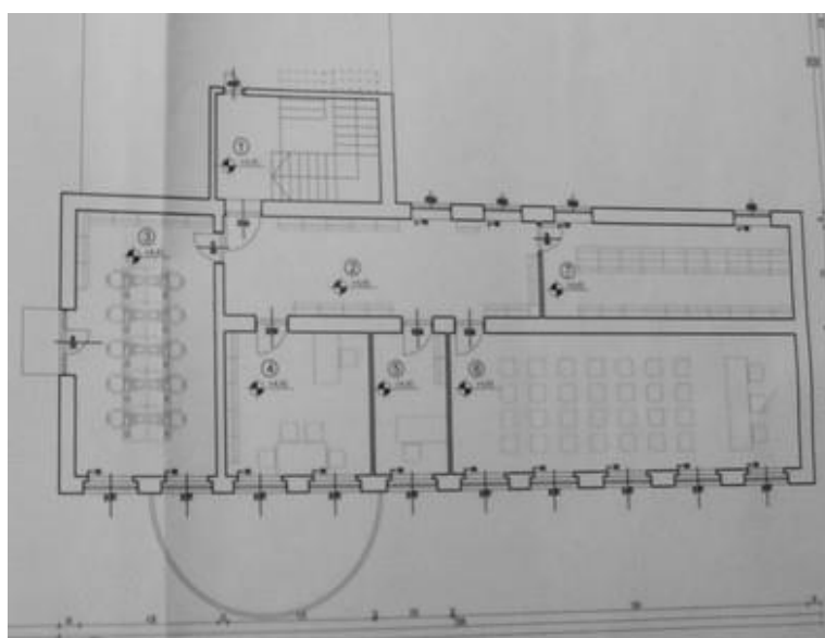
Slika 42. Tlocrt Centra za kulturu Čepin – Knjižnica
